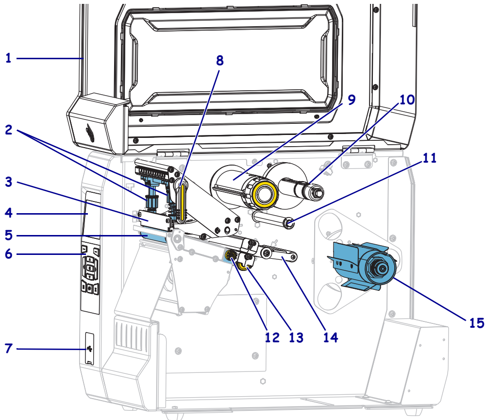
圖 1 • 印表機 零件
