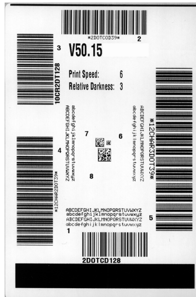
圖 19 • 樣本明暗度和速度測試標籤
