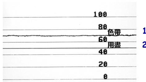
圖 21 • 感應器設定檔 (色帶部份)
