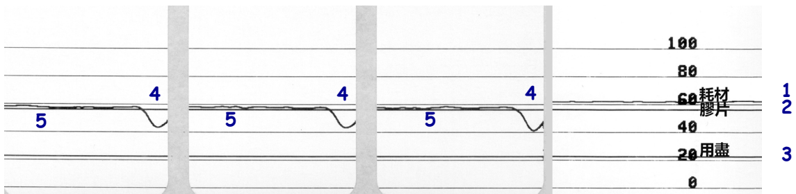
圖 22 • 感應器設定檔 (耗材部份)
