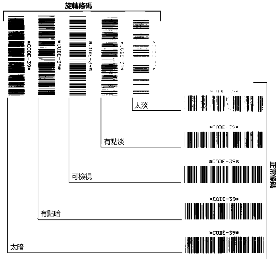
圖 18 • 條碼明暗度比較
