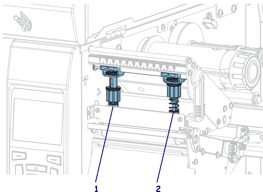
圖 17 • 印字頭壓力插栓
