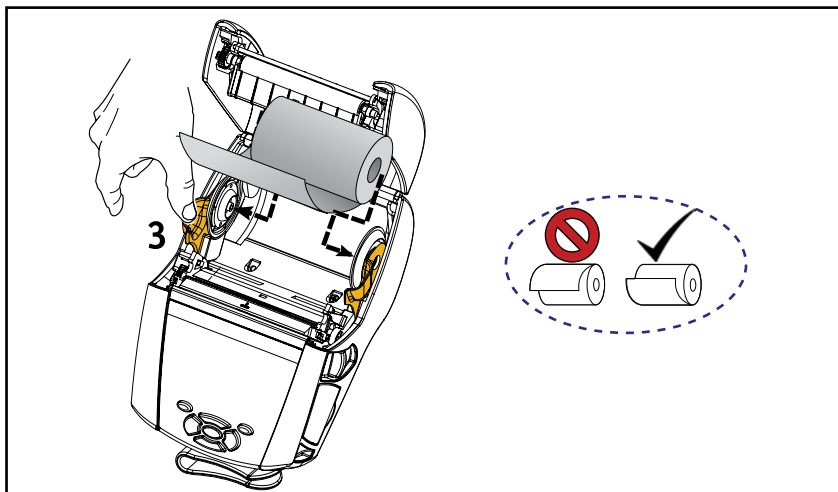
圖 11 • 裝入耗材
