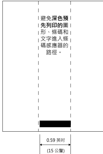
圖 28 • 標籤區域
