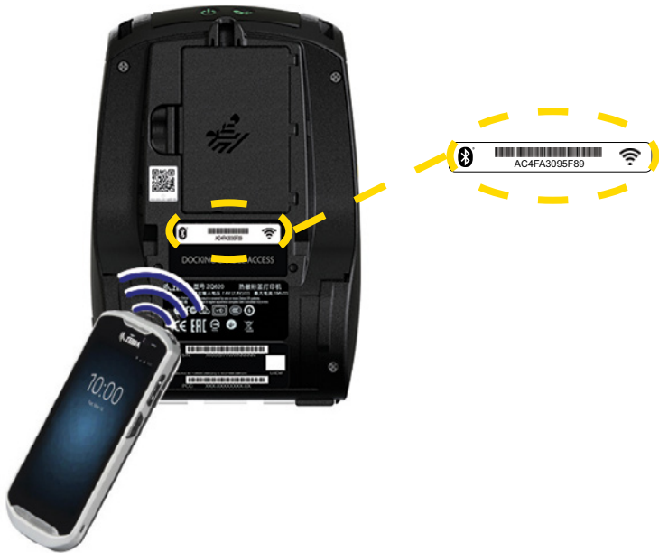
圖 24 • BT/WLAN 通訊
