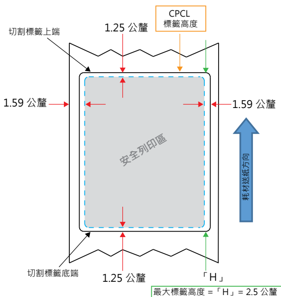
圖 25 • 間隙耗材
